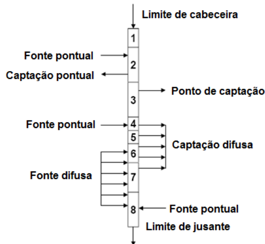
Figura 11 – Diagrama unifilar genérico com o exemplo das entradas.
