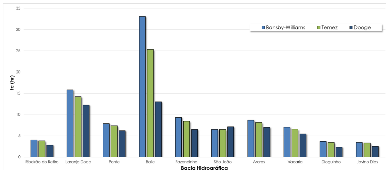
Gráfico 1 - Comparativo do tempo de concentração calculado para as 10 microbacias hidrográficas em estudo.
